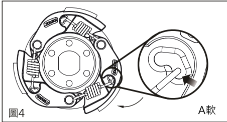
2-1. 小彈簧勾在外側(位置 A)-選擇勾在外側位置時，離合器接合轉速會較低。(圖4)
