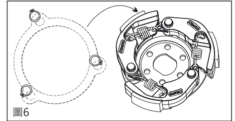
2-3. 裝回內盤鐵片。(圖6)
