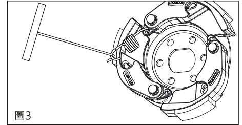
1-3. 先將小彈簧一端固定至孔位，再用彈簧拉柄安裝小彈簧另一端。(圖3)
