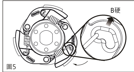
2-2. 小彈簧勾在內側(位置 B)-選擇勾在內側位置時，離合器接合轉速會較高。(圖5)
