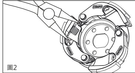
1-2. C型內扣環鉗將小彈簧兩端撐開，安裝至所需孔位，彈簧拉柄。(圖2)
