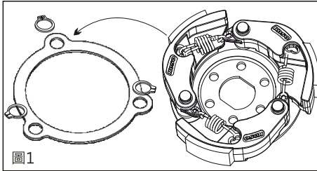
1-1. 使用工具，先取下內盤鐵片。(圖1)
